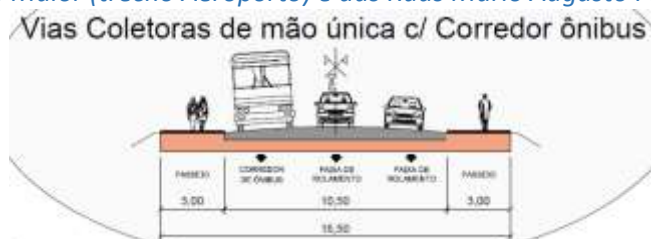
Seção da Domingos Mafrense à intersecção em rótula
