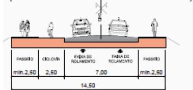
Seção da Rua Manoel Aguiar Filho ("Av. Hiroshima")
