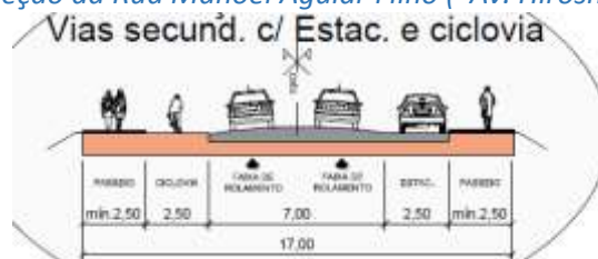
Seção da Av. Mestre João Isidoro da Fonseca
