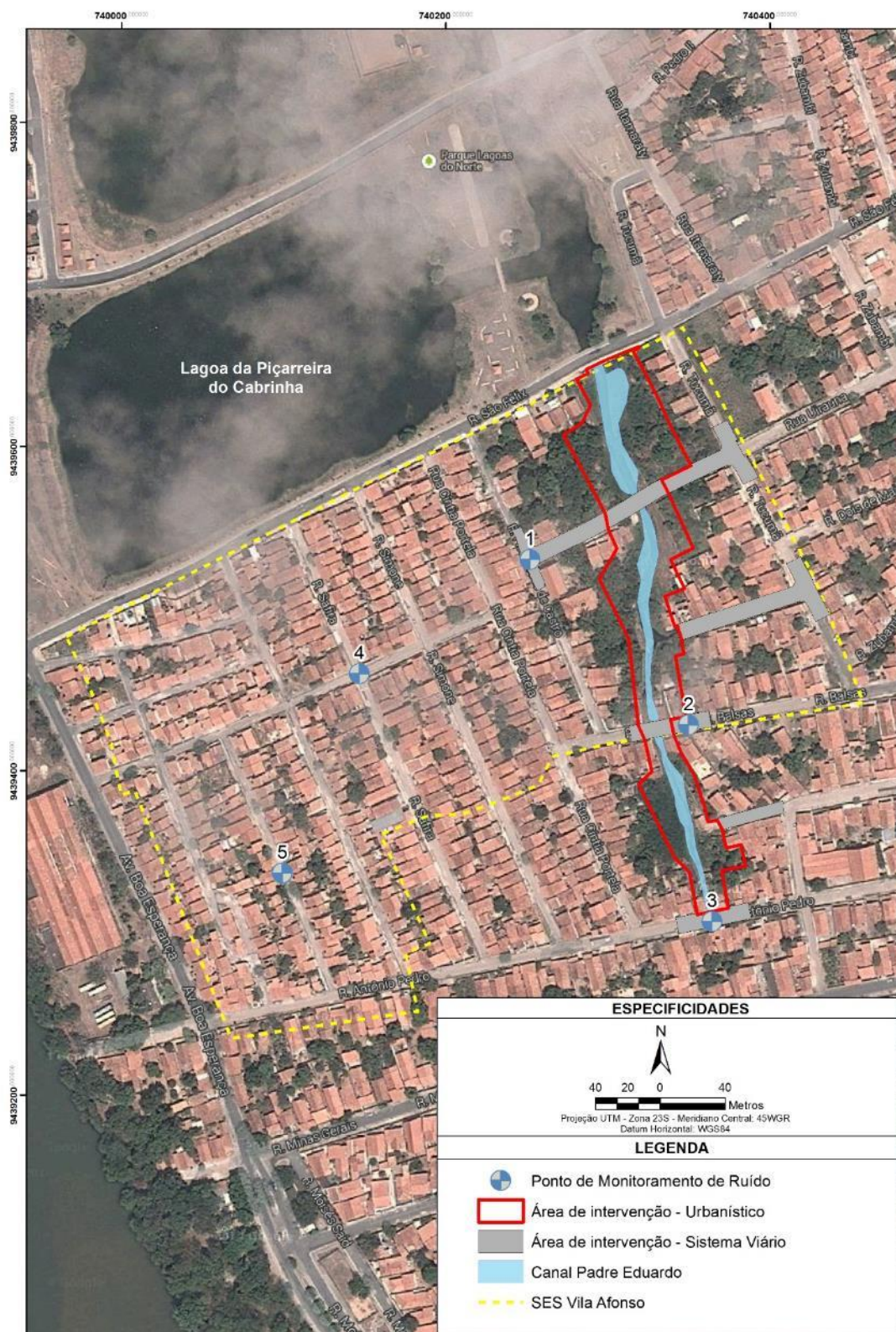
Figura 65. Monitoramento de Ruído.
