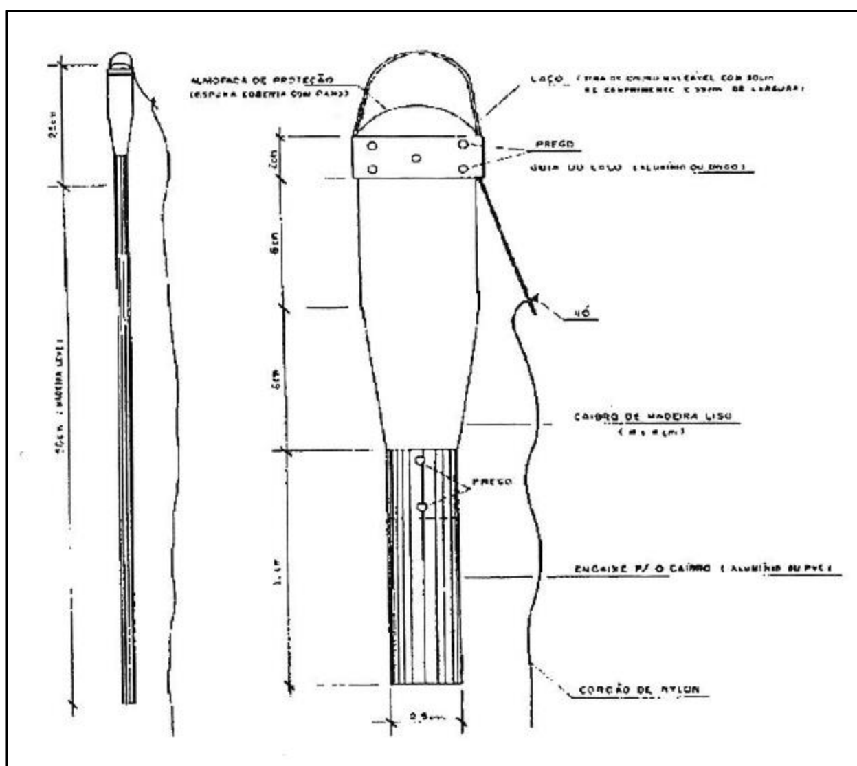
Figura 73. Modelo de Laço de lutz para captura de serpentes.
