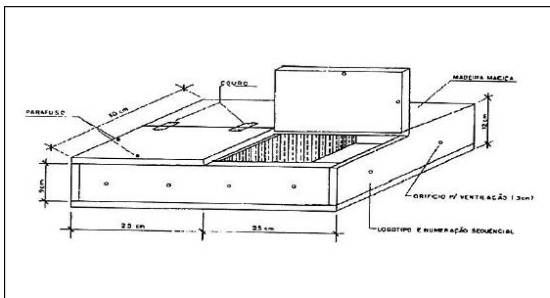
Figura 75. Caixa para transporte de ofídios – modelo Butantã.
