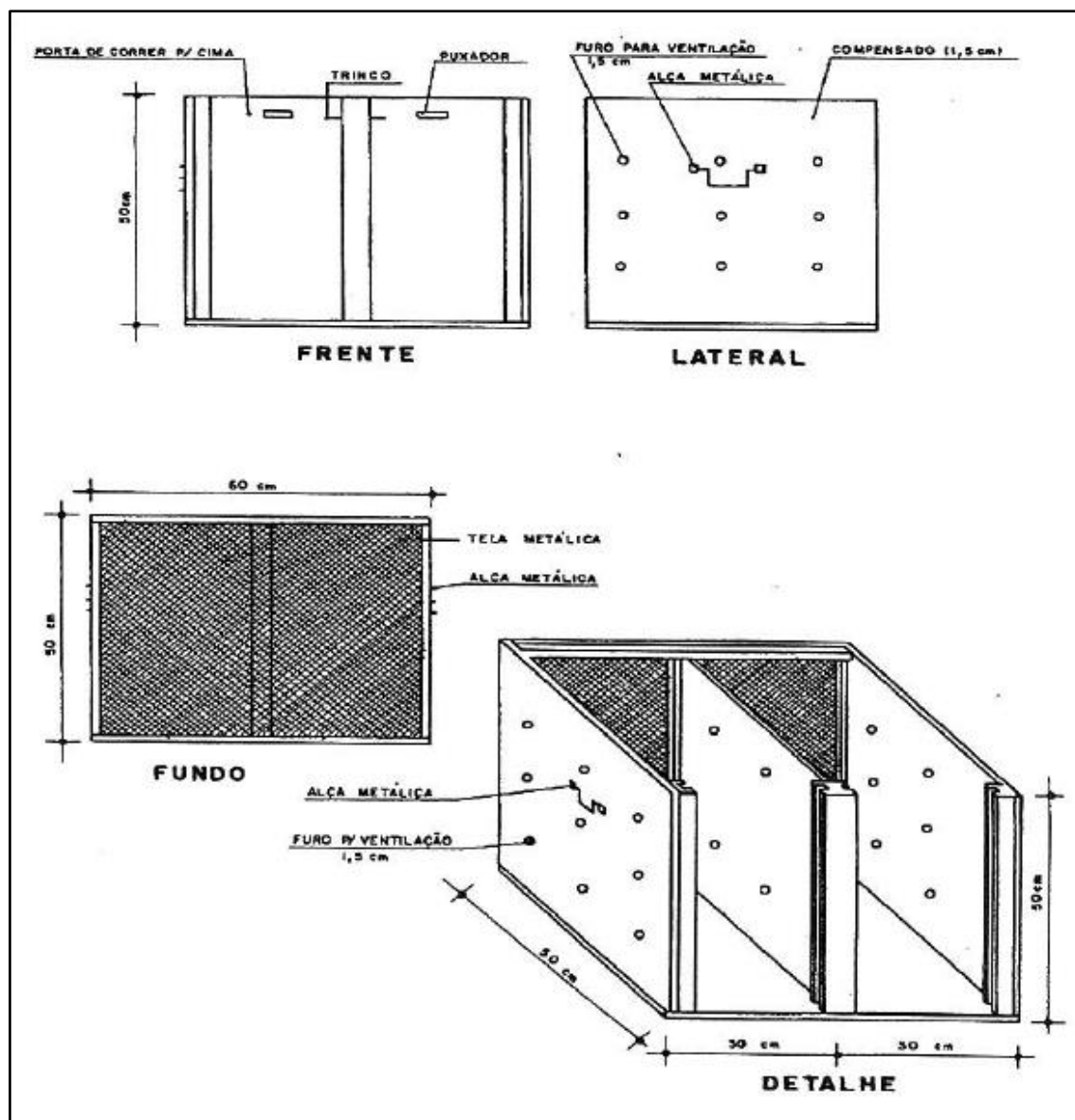
Figura 77. Caixa de transporte de animais de pequeno porte.
