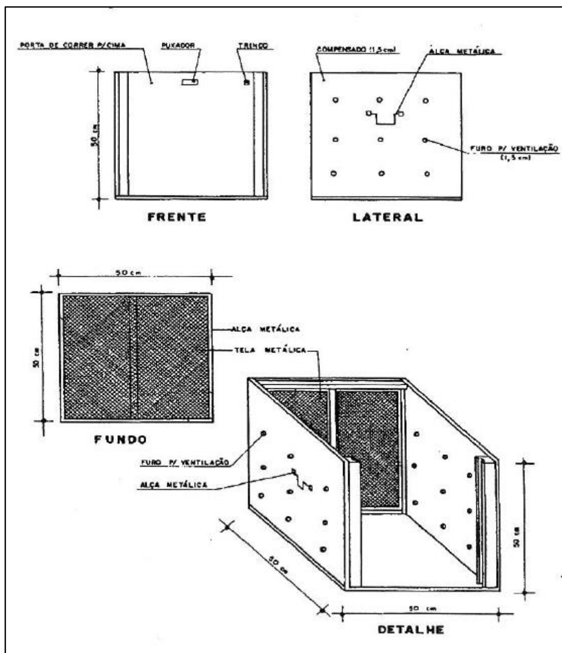
Figura 78. Caixa de transporte de animais de médio porte.
